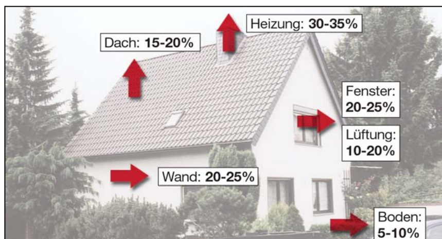
Typische Wärmeverluste eines Einfamilienhauses (Quelle: BINE Informationsdienst, Bonn)
